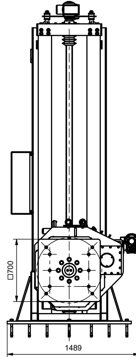
A-A ( 1 : 25 ) Master
